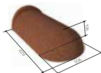
GĄSIOR POCZĄTKOWY 205
