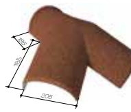
TRÓJNIK GĄSIORA 205 30-45°
